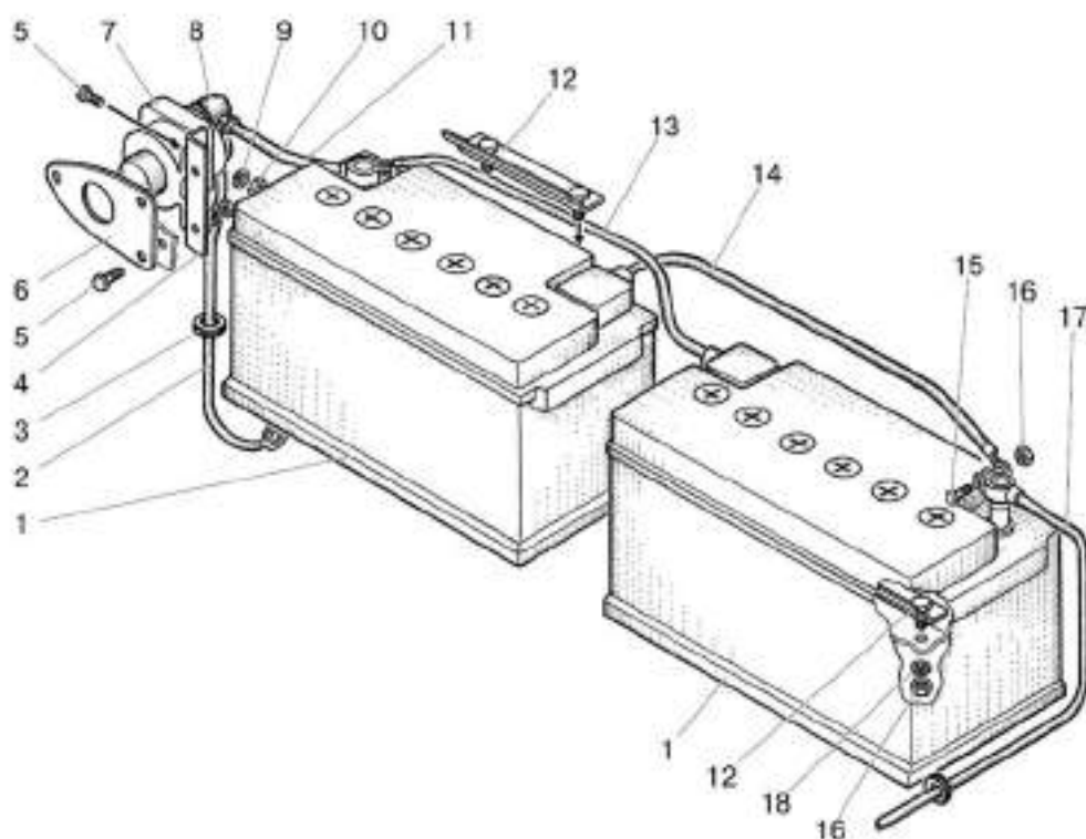
Мал. 37.4. Батареї акумуляторні. Встановлення акумуляторних батарей із системою запуску 12В. (крім трактора «БЕЛАРУС-82П»)
