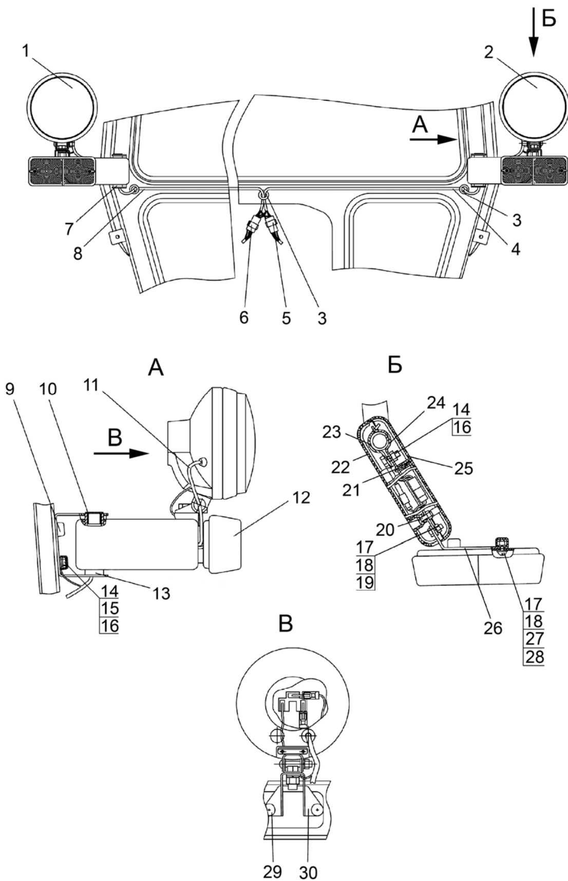
Мал. 37.16. Встановлення ліхтарів передніх з дорожніми фарами (для трактора «БЕЛАРУС-82П»)
