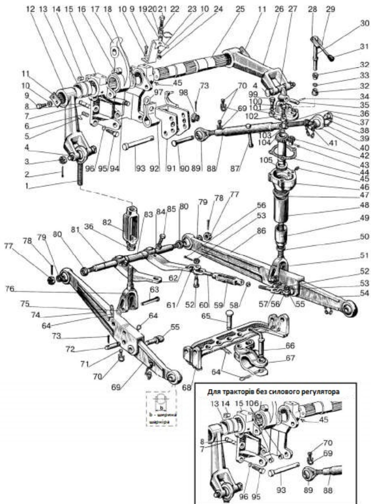
Мал. 46.1. Механізм задньої навіски (для тракторів із силовим регулятором та без силового регулятора)
