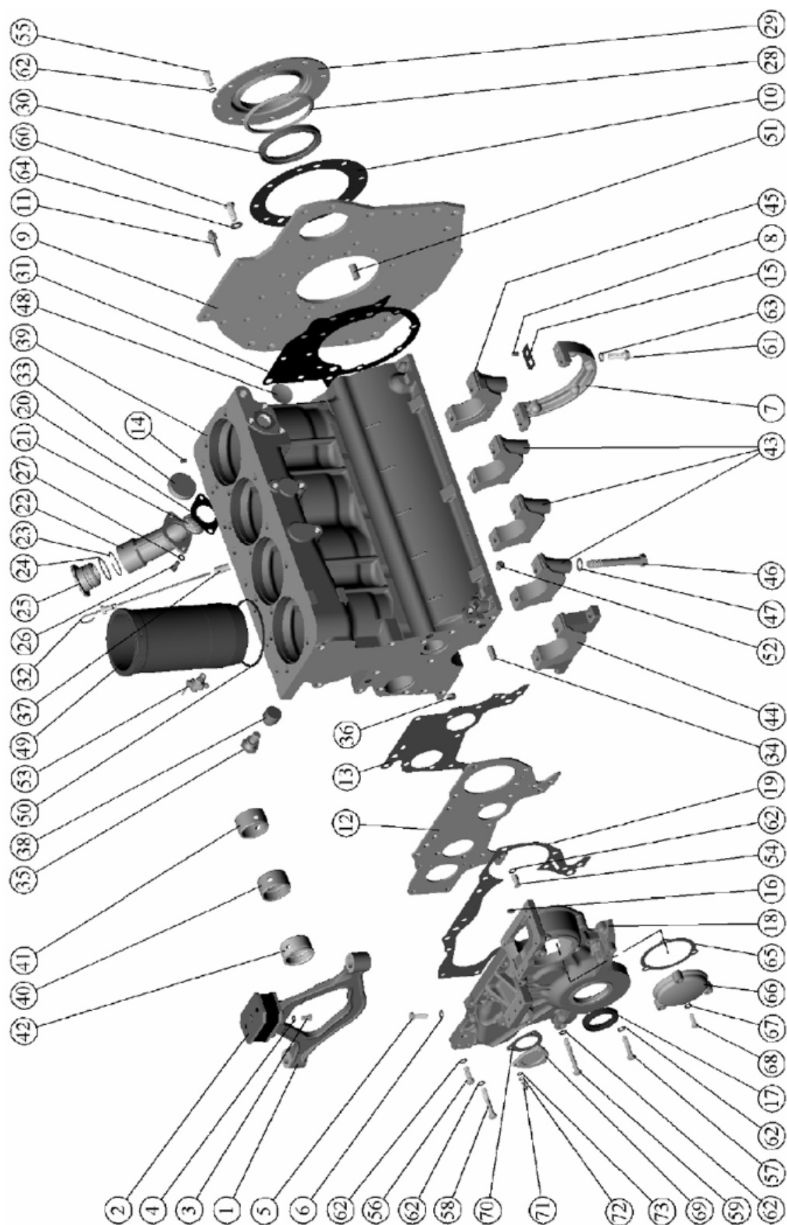
Мал. 10.1. Підвіска та блок циліндрів
