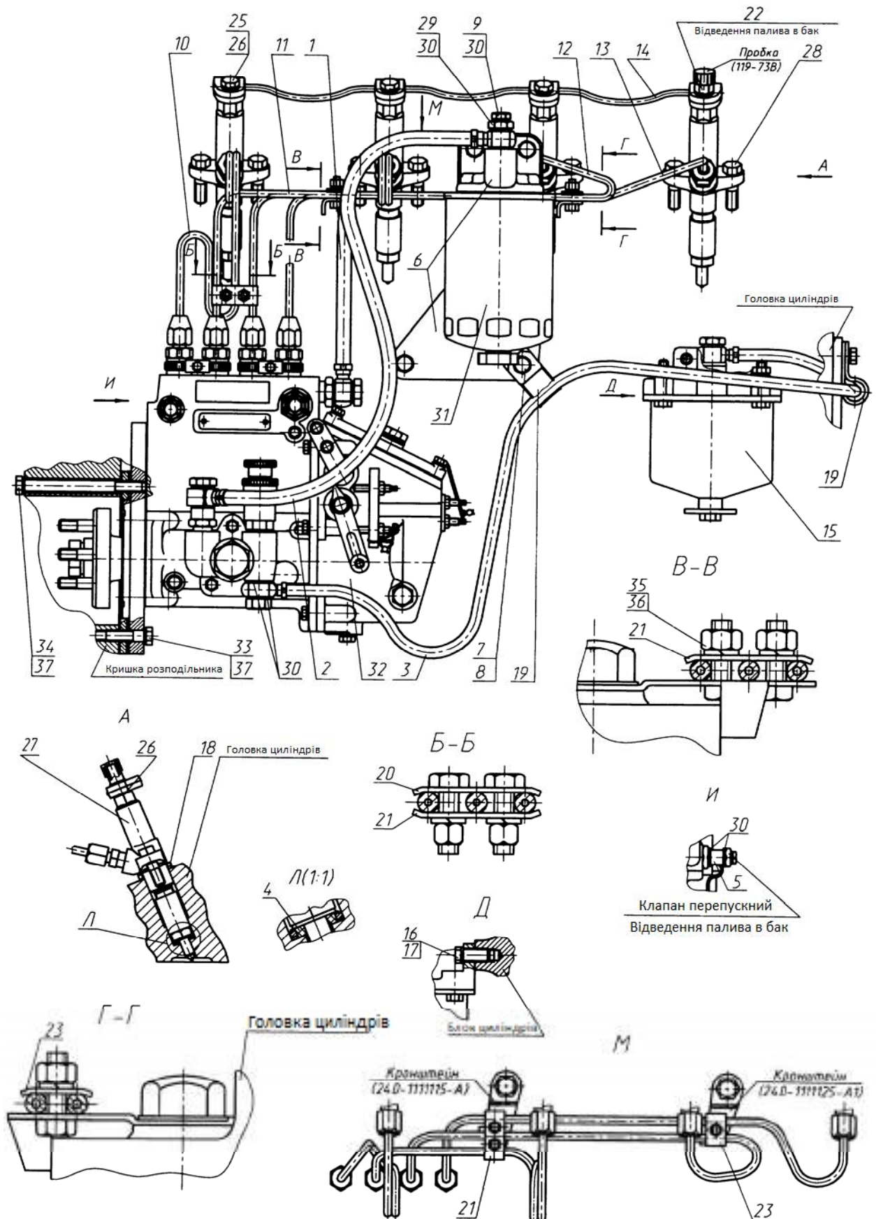
Мал. 11.6. Паливна апаратура (для двигуна Д-243С з паливним насосом виробництва ВАТ «НЗТА»)
