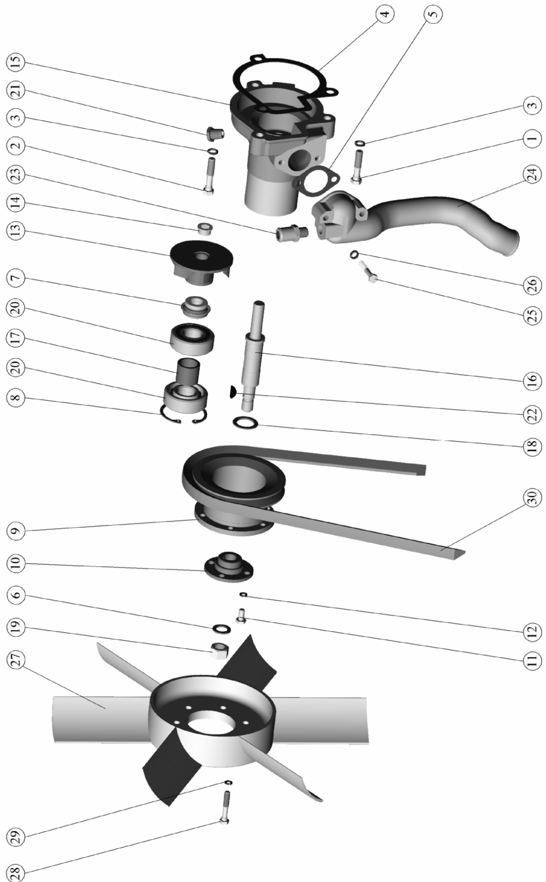
Мал. 13.3. Насос водяний та вентилятор
