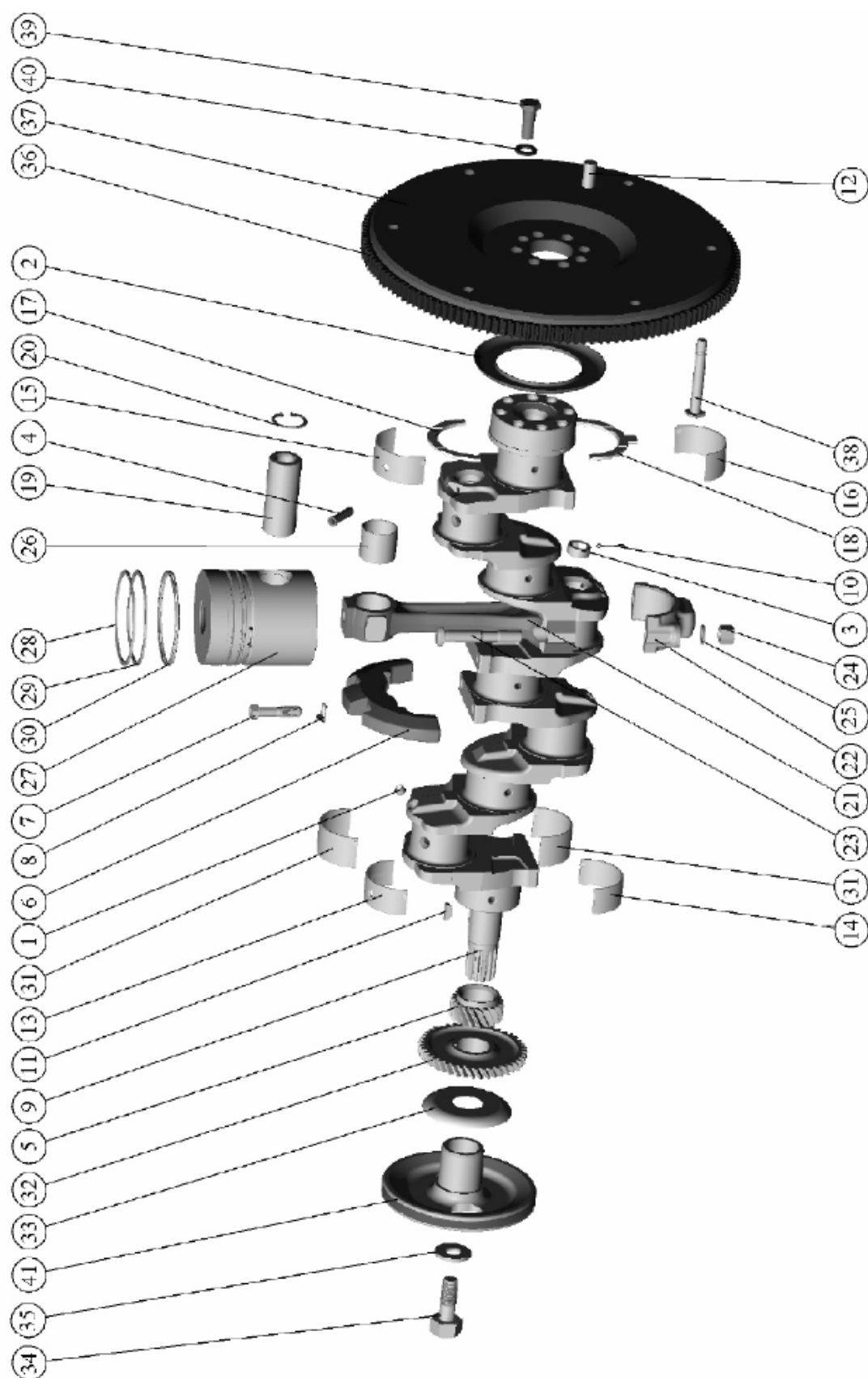
Мал. 10.3. Поршні та шатуни. Вал колінчастий та маховик
