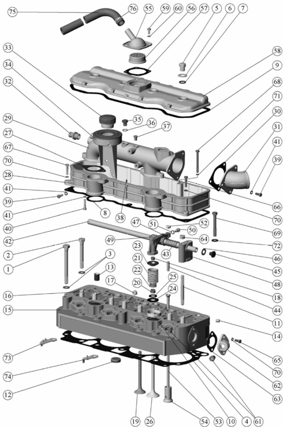
Мал. 10.2. Головка циліндрів. Клапани та штовхачі клапанів
