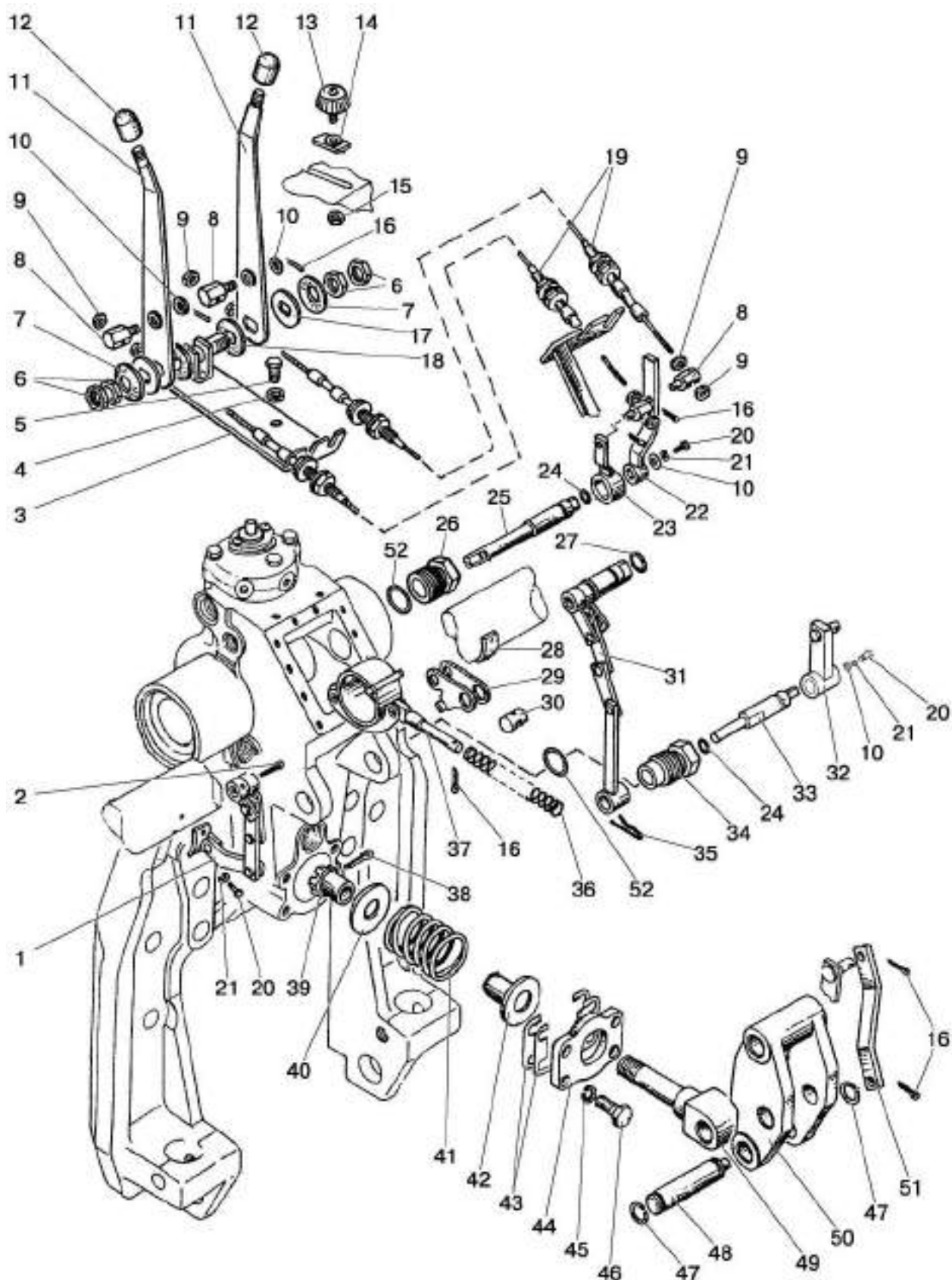
Мал. 46.28. Гідропідійомники. Управління гідропідійомником (Для трактора «БЕЛАРУС-82П» з гідропідійомом)
