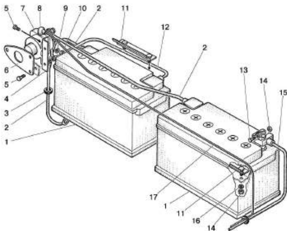
Мал. 37.4. Батареї акумуляторні. Встановлення акумуляторних батарей із системою запуску 12В. (крім трактора «БЕЛАРУС-82П»)
