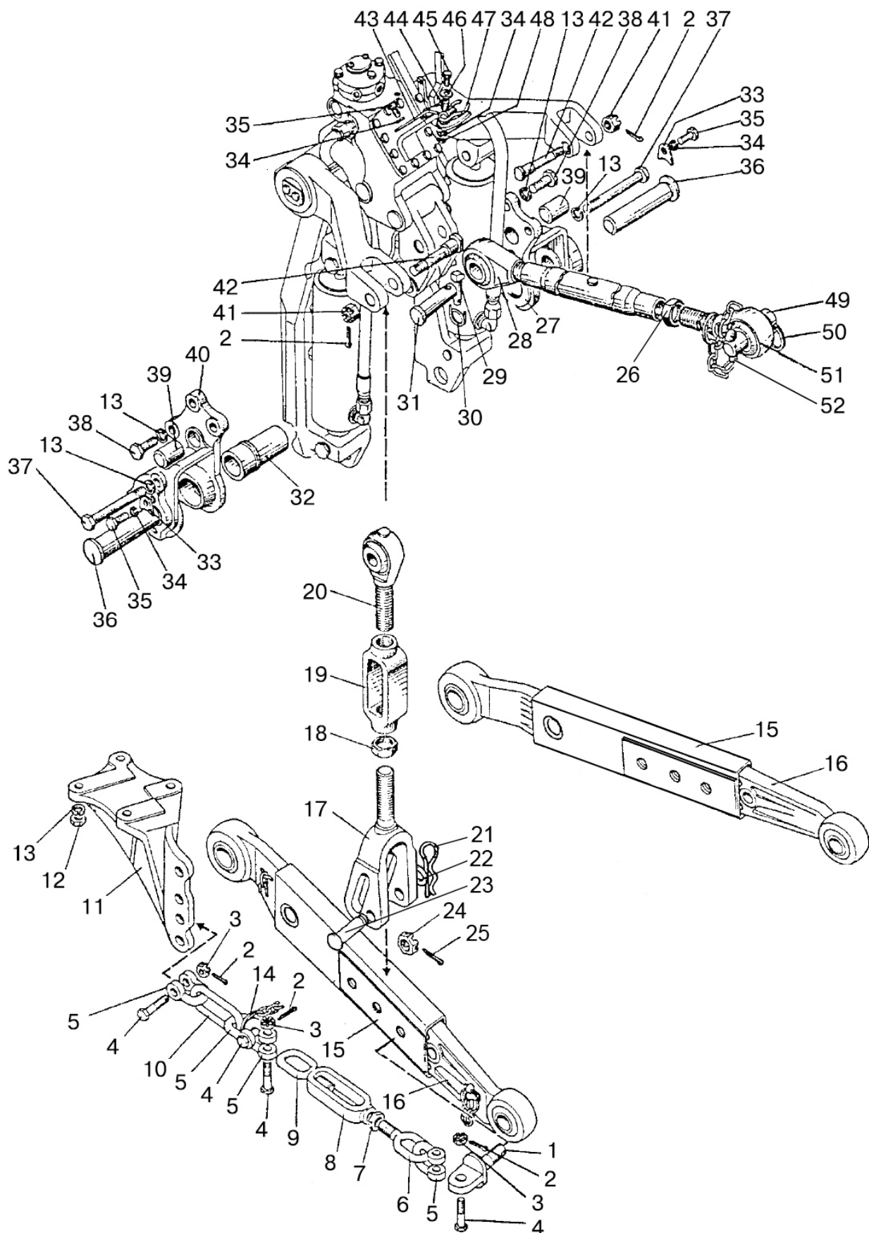
Мал. 46.2. Механізм задньої навіски (варіант для трактора «БЕЛАРУС-82П» з гідропідйомником)
