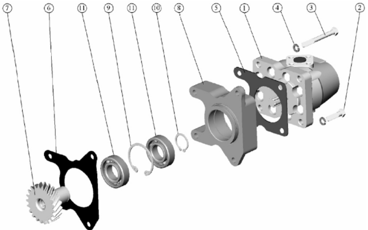
Мал. 10.6. Насос рульового керування
