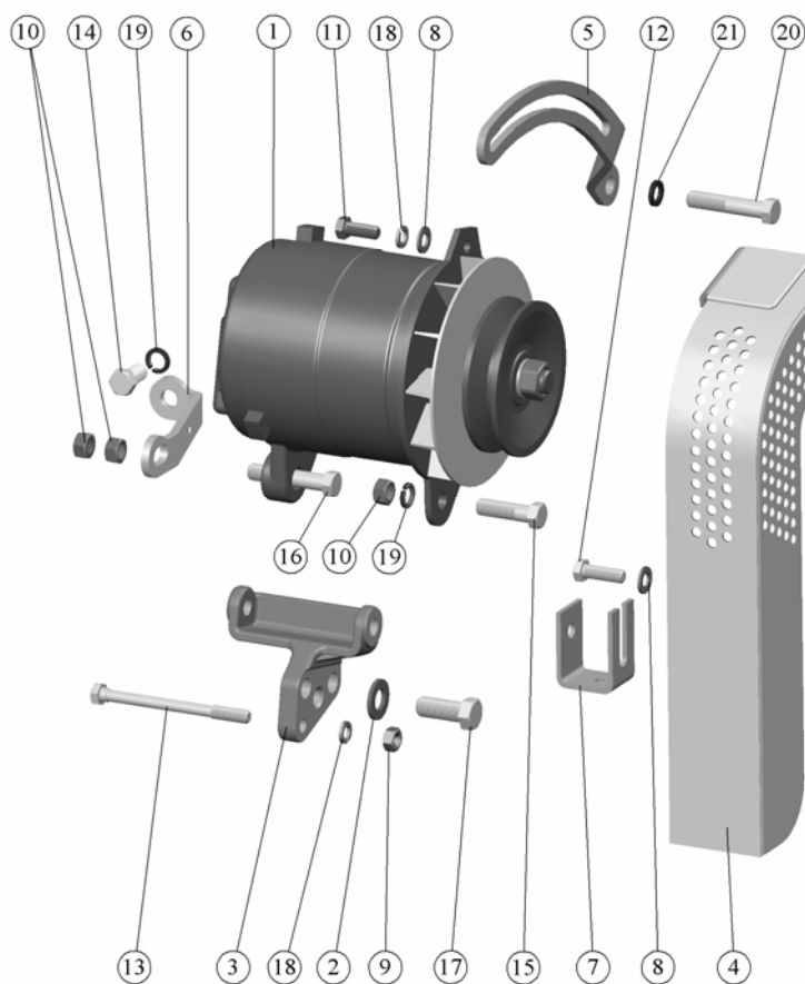
Мал. 37.8. Генератор (для трактора «БЕЛАРУС-80.3/82.3»)
