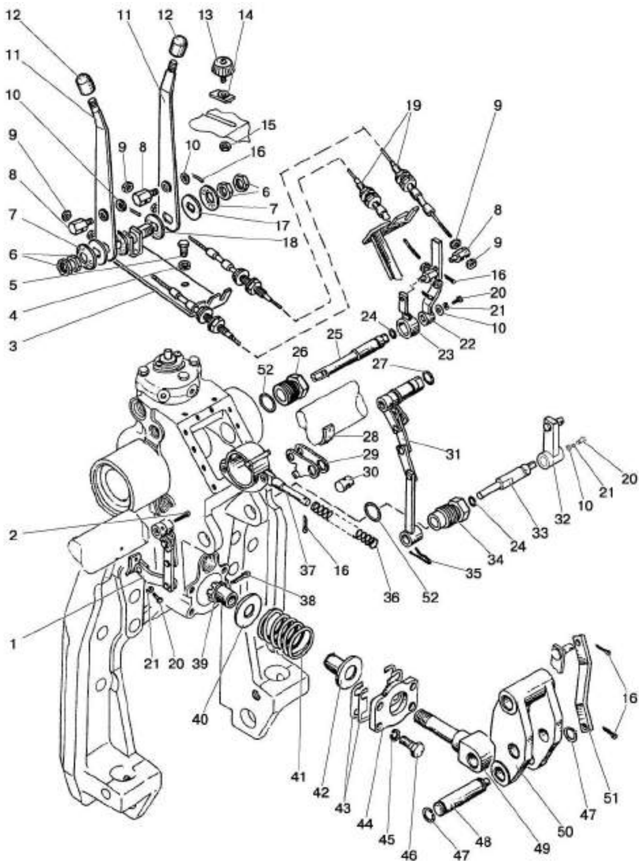
Мал. 46.28. Гідропідйомники. Управління гідропідйомником (Для трактора «БЕЛАРУС-82П» з гідропідйомом)
