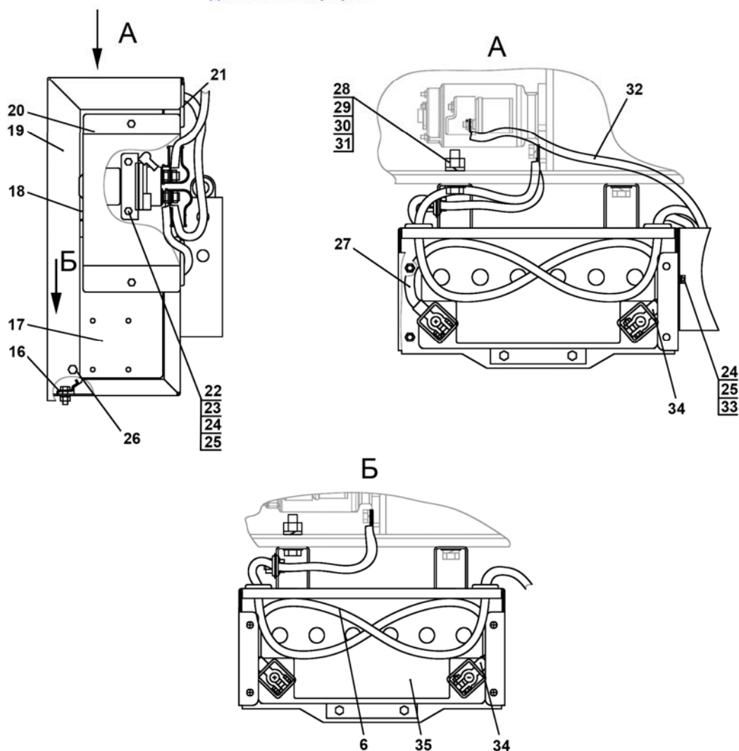
Мал. 37.6. Батареї акумуляторні. Встановлення акумуляторних батарей. (Для трактора «БЕЛАРУС-82П»)
