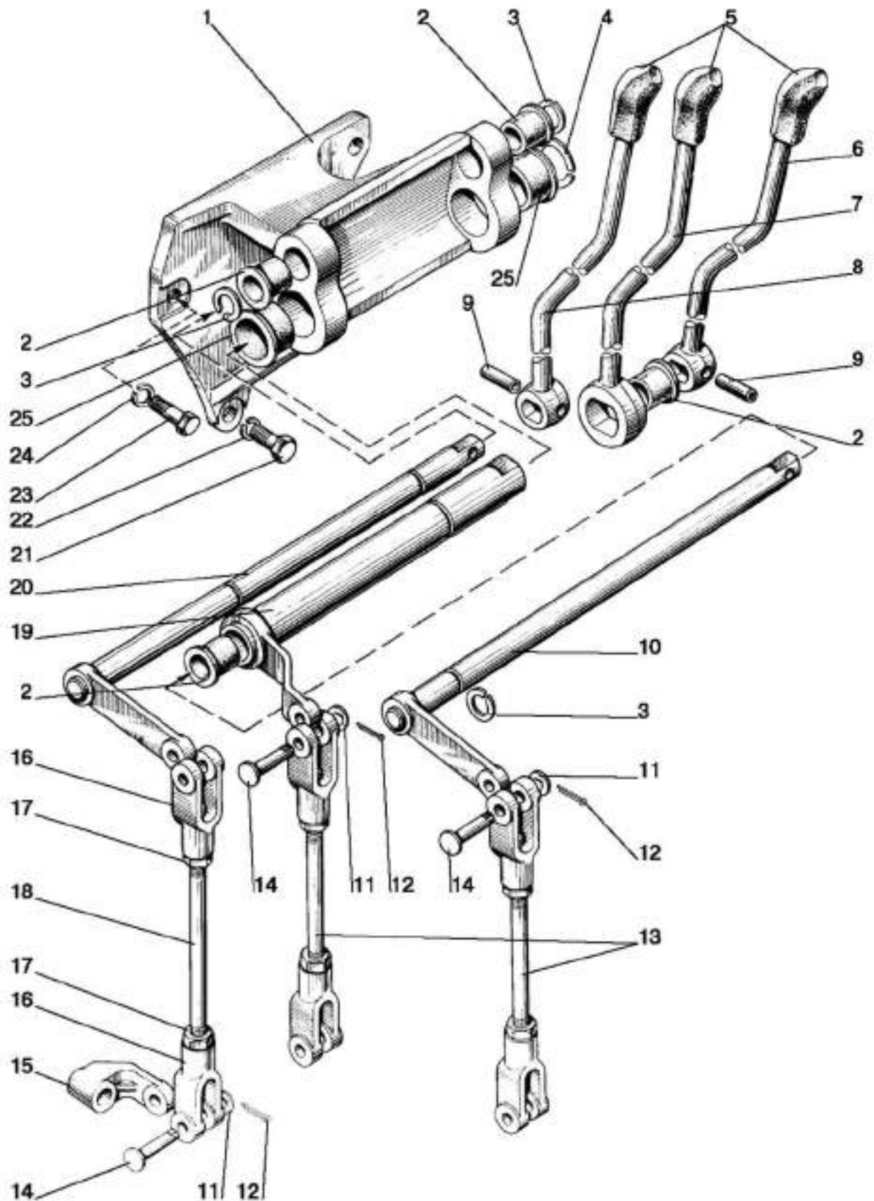
Мал. 46.4. Управління гідророзподільником (для тракторів з силовим регулятором та без силового регулятора)
