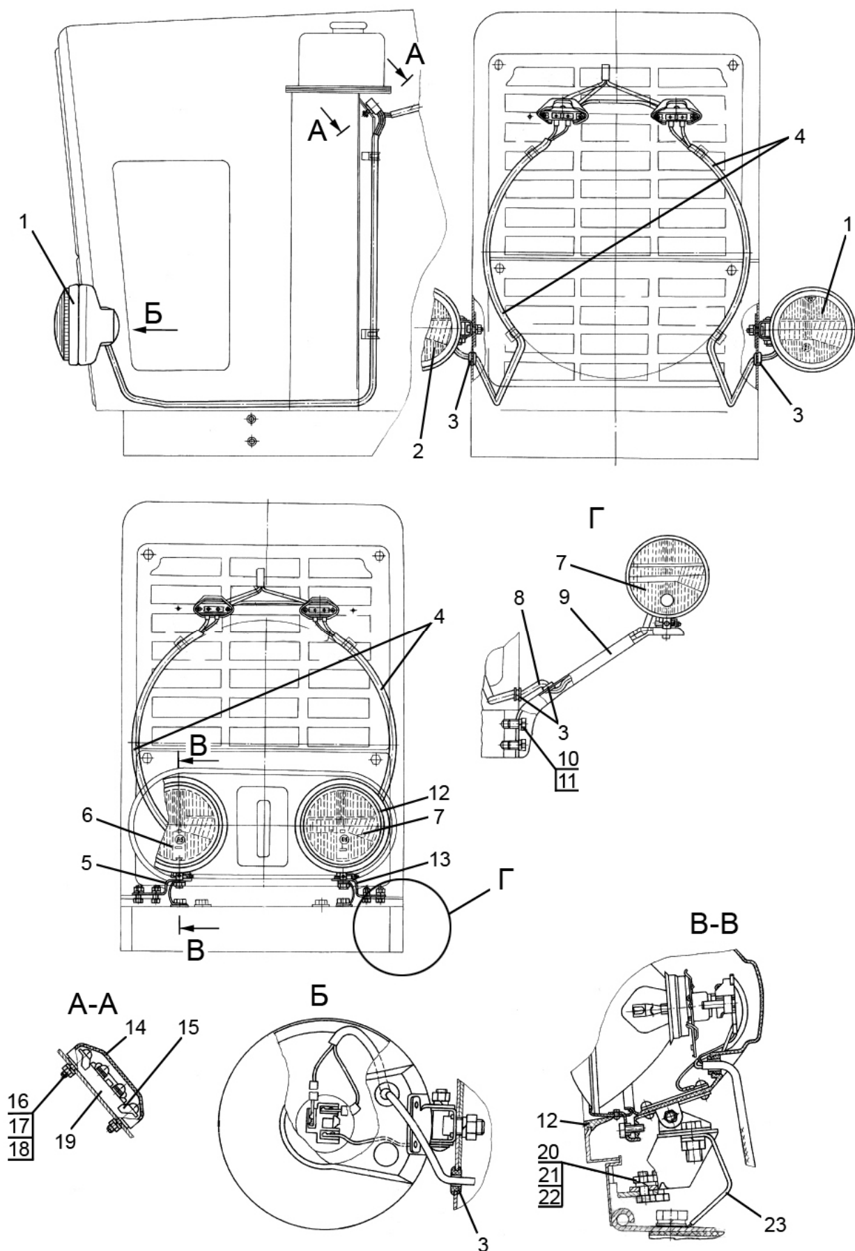
Мал. 37.15. Встановлення фар дорожніх
