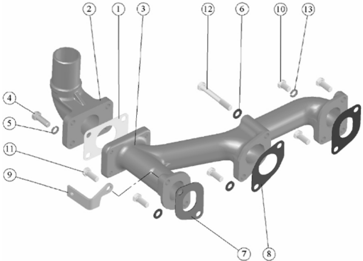
Мал. 10.5. Випускний колектор
