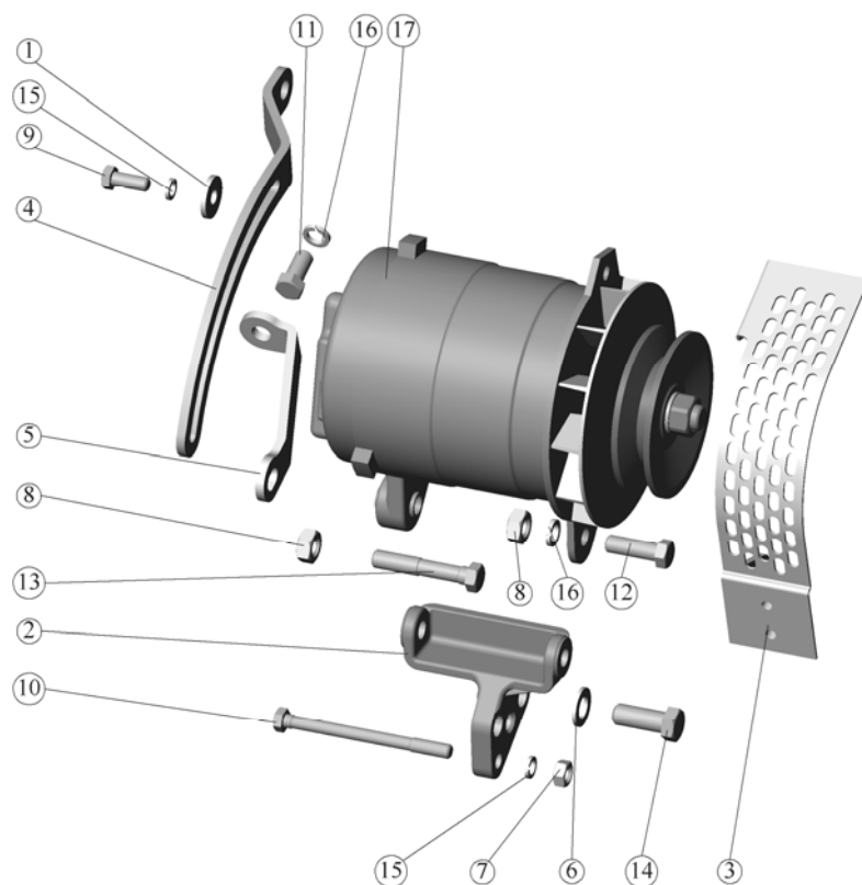
Мал. 37.7. Генератор (для трактора «БЕЛАРУС-80.1/80.У/82У/82.1/820/82Р/82П»)
